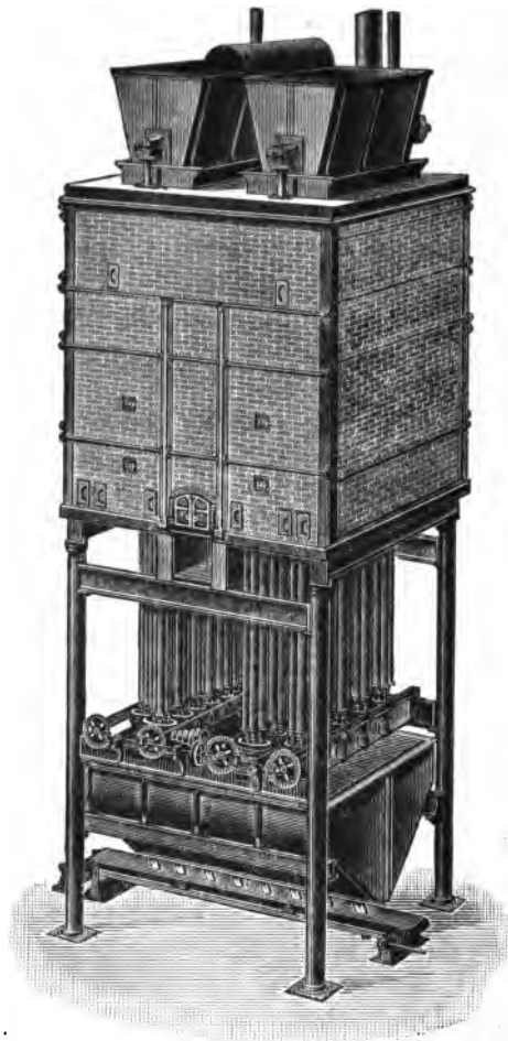
FIG. 37.—CHAR PIPE-KILN
